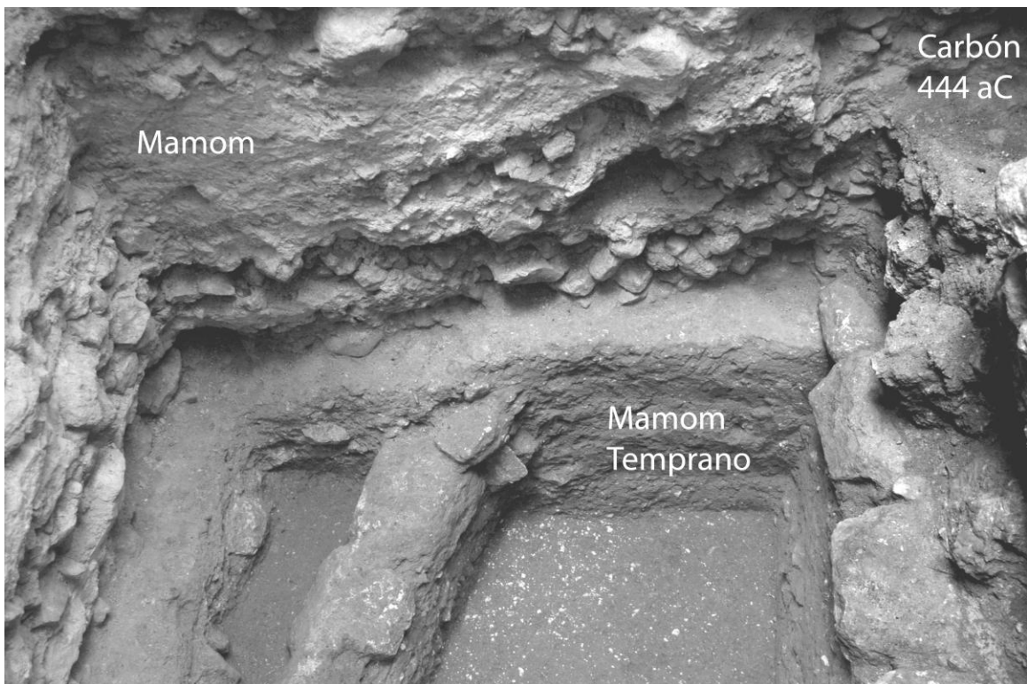
Figura 9 Perfil Norte de Estructura 1 de Anonal, mostrando niveles tempranos.
